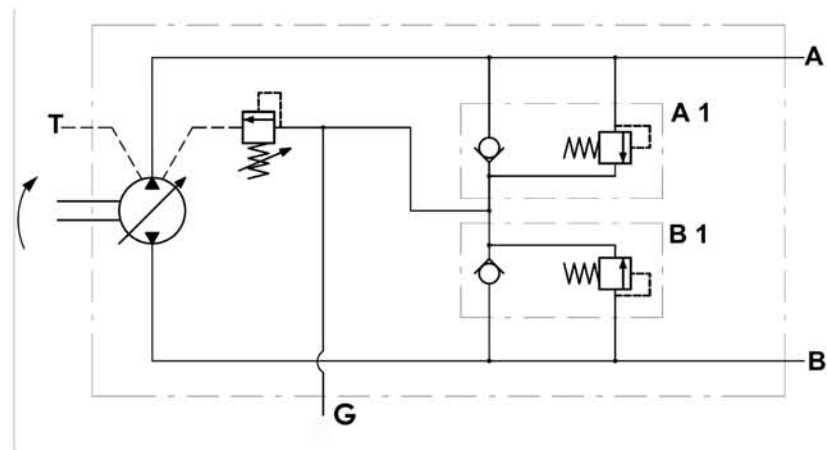
液压原理图
